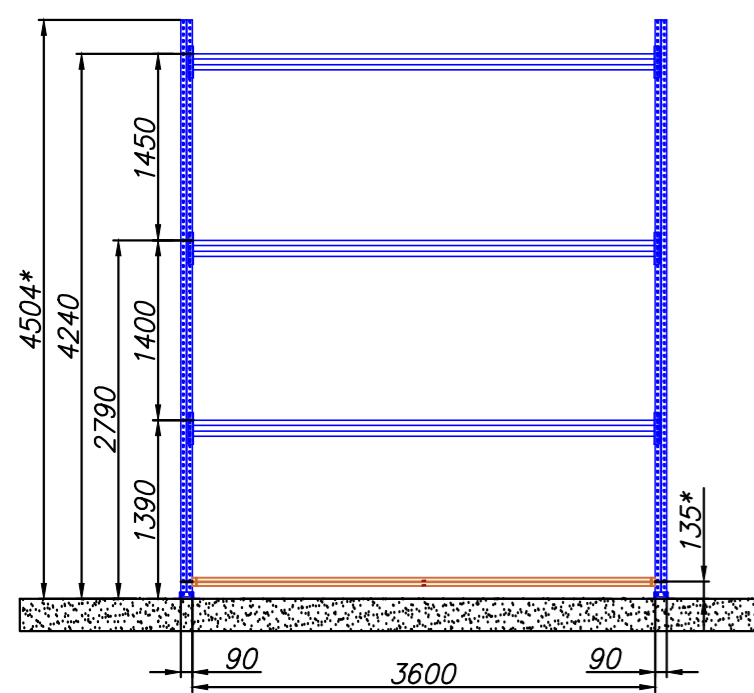
Установка паллетостопов (Ряд 1)
