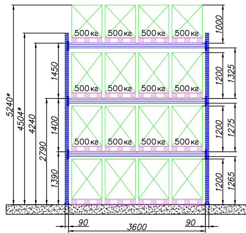
Установка паллетостопов (Ряд 1)
