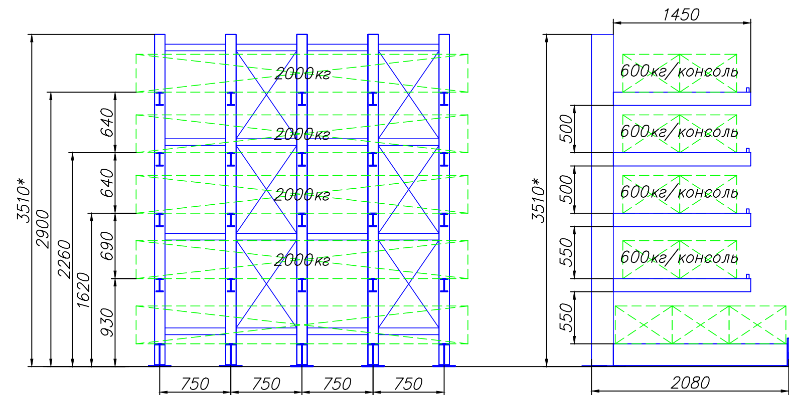
Консольный стеллаж для хранения пачек профиля Вместимость пачек профиля: 22 п/м.
