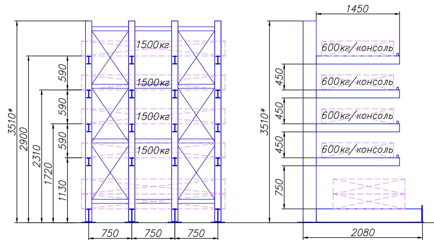
Консольный стеллаж для хранения листов Вместимость листов на поддоне: 18 п/м.
